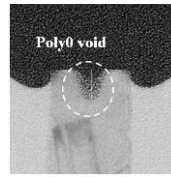
Fig.9. Poly0 void TEM cross-section
