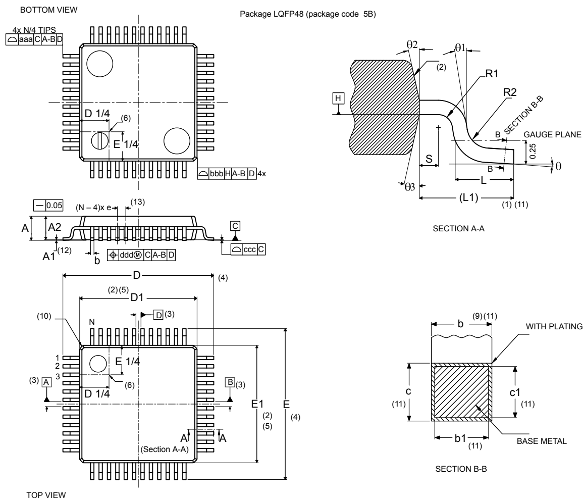
Figure 47. LQFP48- Outline (15.)
