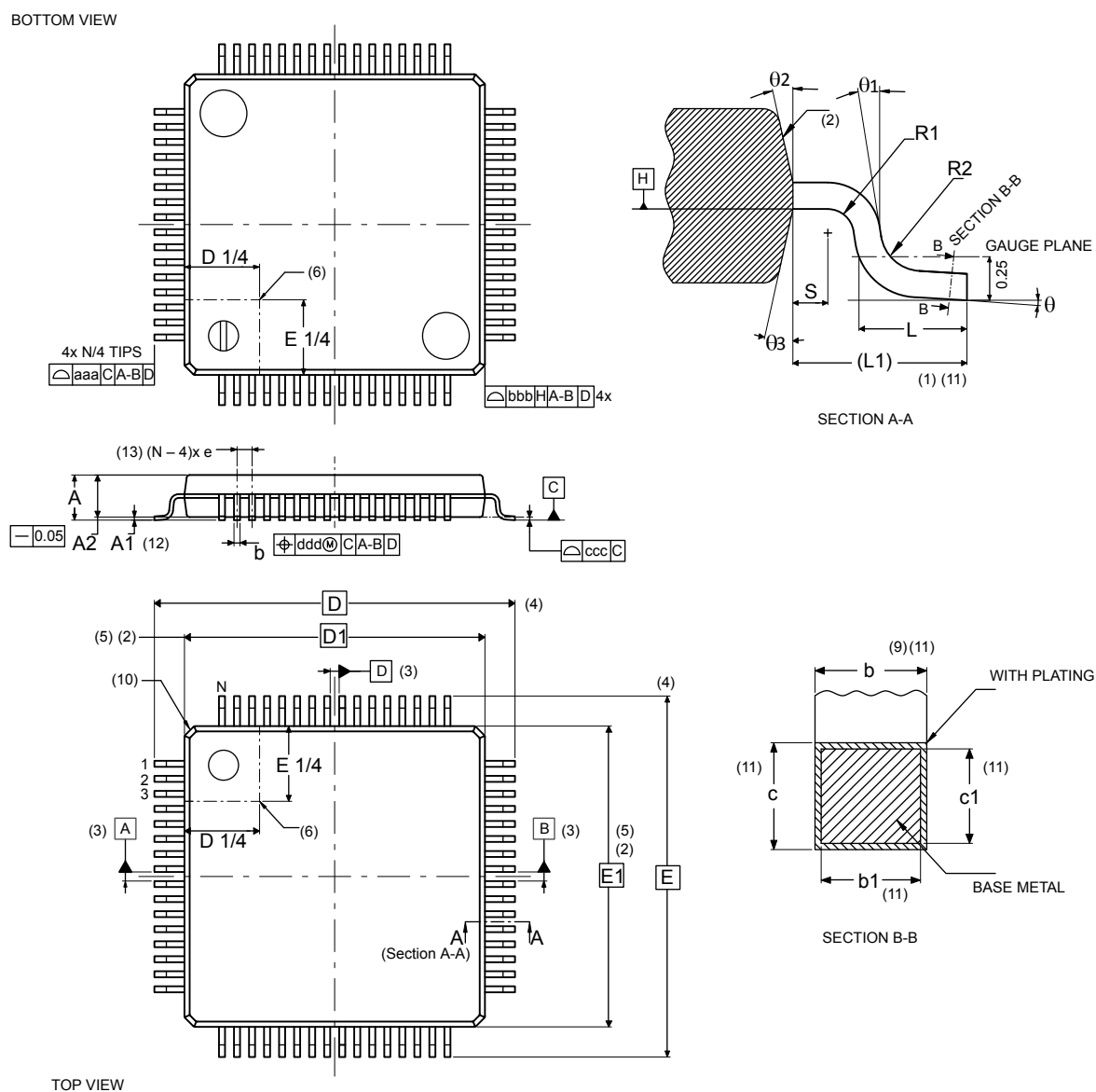
Figure 45. LQFP64 - Outline (15.)
